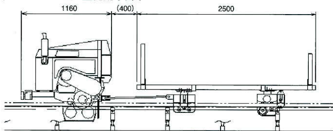
動力車 KS-200型+重荷用台車 DJ-20(4人乗用)
