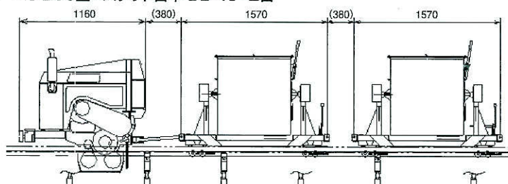
動力車 KS-200型+バケット台車 DB-40×2台
